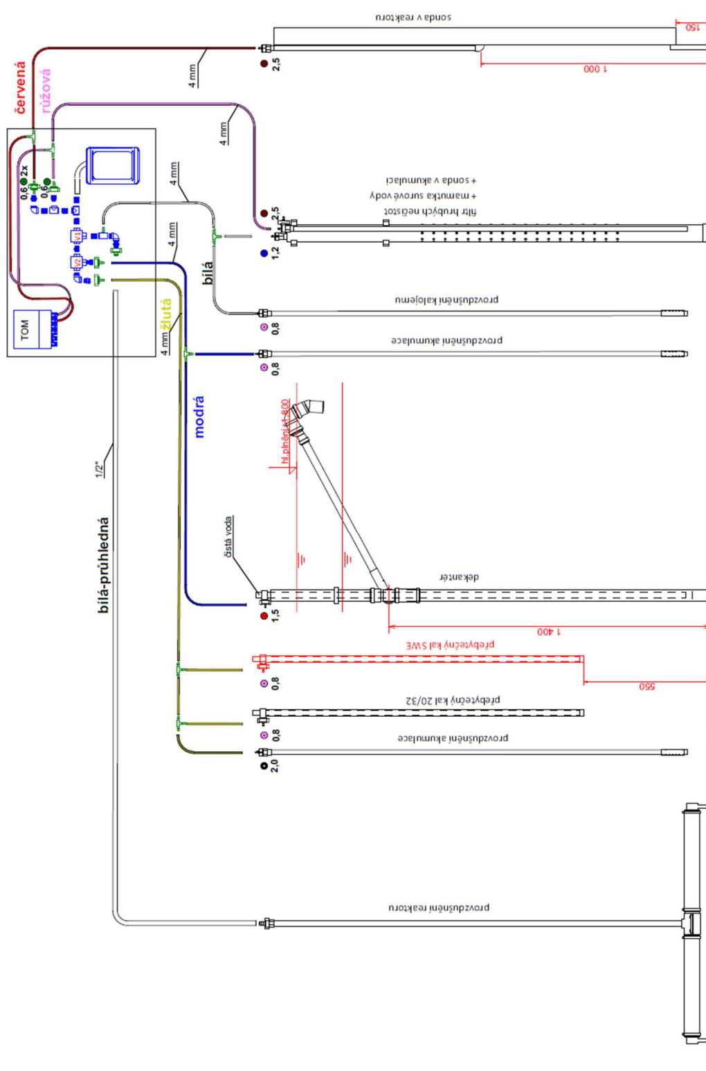
Obrázek 11: Schéma rozvodů vzduchu TOPAS S 10
